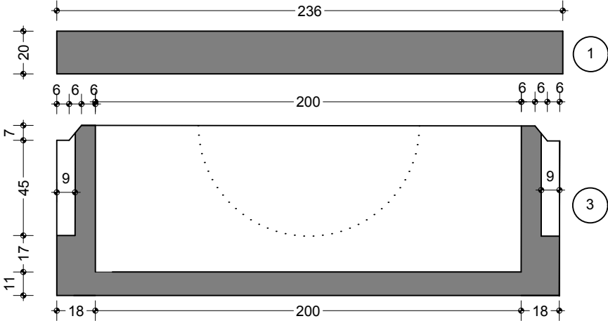
SEZIONE POZZETTO A-A SCALA 1:25
