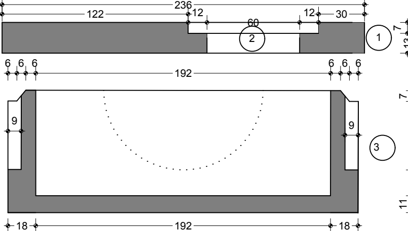
SEZIONE POZZETTO B-B SCALA 1:25
